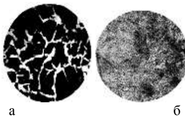
Микроструктуры углеродистой отожженной стали с различным содержанием углерода (×300)
