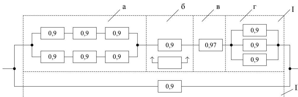
Рис.1. Схема расчета надежности.
