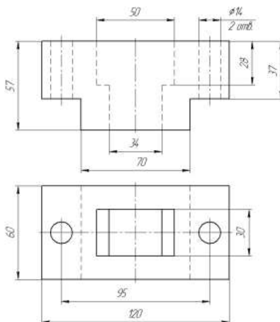
Образец типовых вариантов заданий 4 и 5 РГР (3 КР) по теме «Соединения резьбовые»
