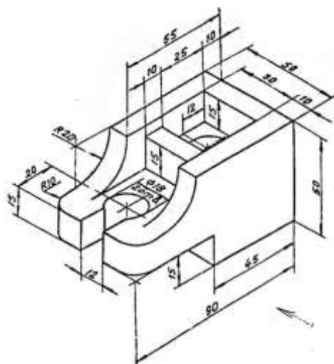
Образец типового варианта задания 3 РГР по теме «Прямоугольная изометрия»
